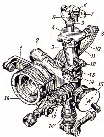
Рис. 3. Прицел для не прямой наводки: 1 — цапфа коробки прицела; 2 — коробка прицела; 3 — корзина для панорамы; 4 — панорама; 5 — головка; 6 — барабан отражателя; 7 — визир; 8 — барабан угламера; 9 — кольцо угламера; 10 — орудийная стрелка; 11 — стрелка прицела; 12 — окуляр; 13 — поперечный уровень; 14 — боковой уровень; 15 — маховик; 16 — тайка подъёмного механизма прицела; 17 — шкала углов места цели; 18 — дистанционный барабан.
